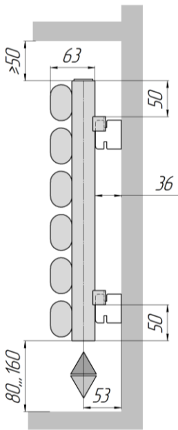
ELLIPSE S H 1 (вид сбоку, для n > 4 , кронштейны КС 22)
