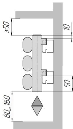
ELLIPSE S H 1 (вид сбоку, для n=3 , кронштейны КС 22)
