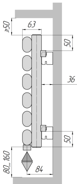
ELLIPSE S H 1 R (вид сбоку, для n>4, кронштейны КС 22)
