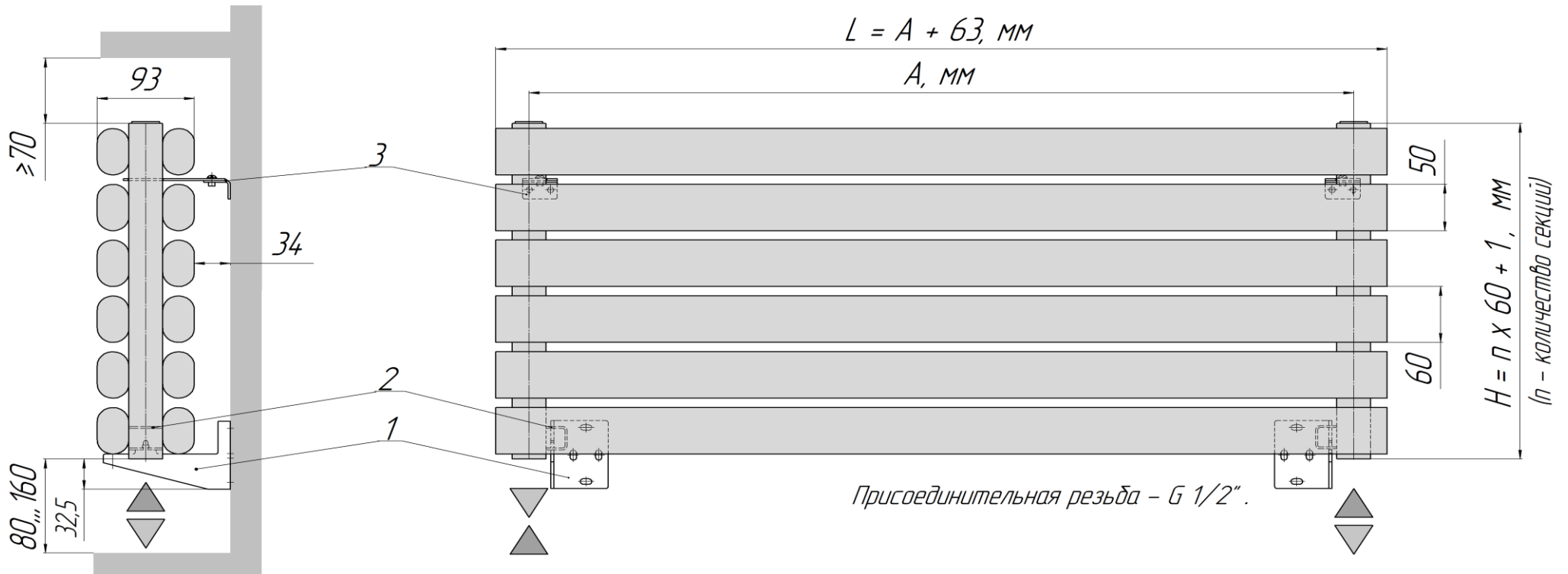
ELLIPSE S H 2 (вид сбоку, крепления комплект №1)
