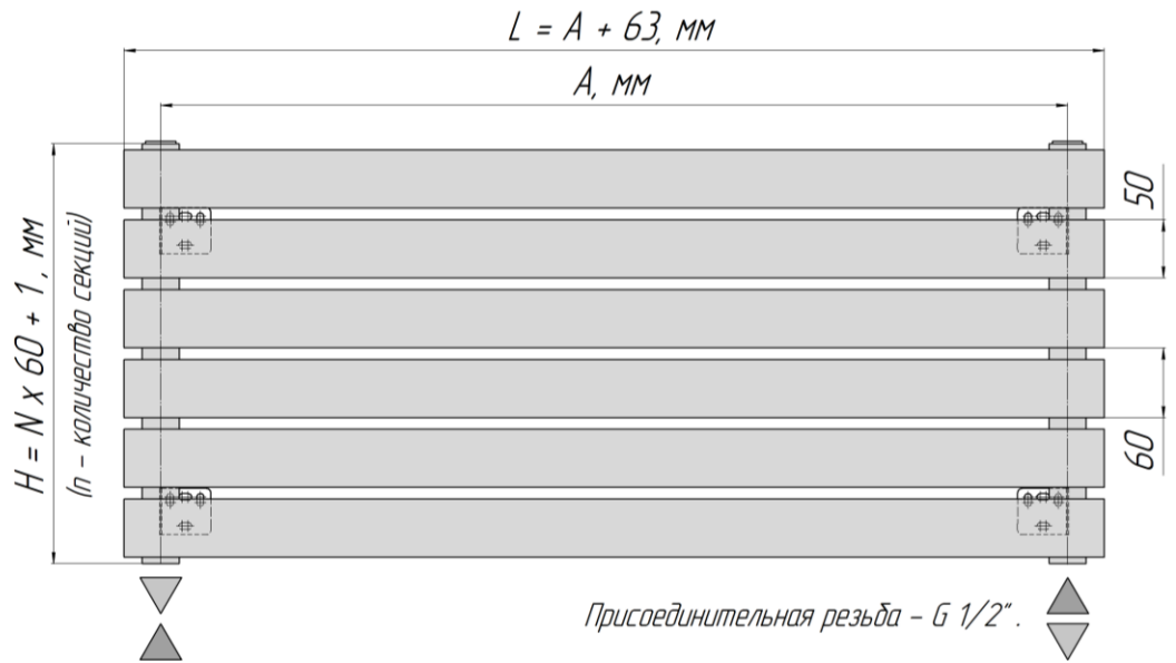
ELLIPSE S H 1 (вид сверху)
