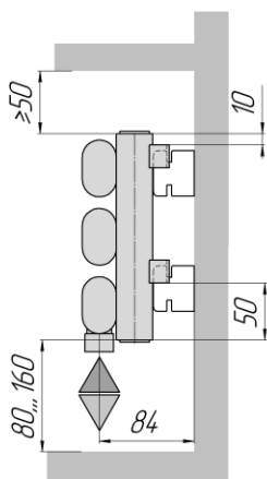
ELLIPSE S H 1 R (вид сбоку, для n=3, кронштейны КС 22)
