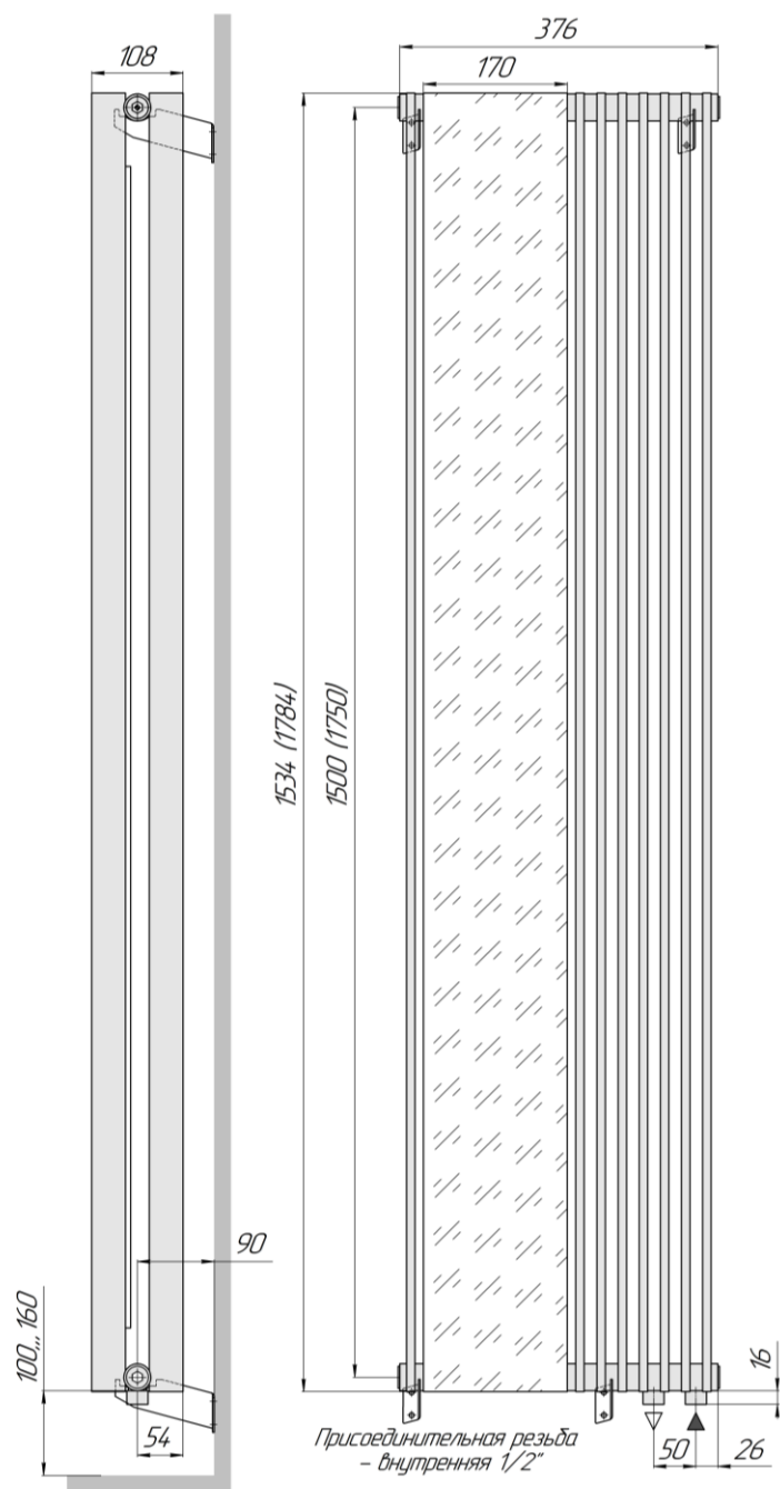
Зеркало П 2-1-7 (вид сбоку, кронштейны КР-90)
