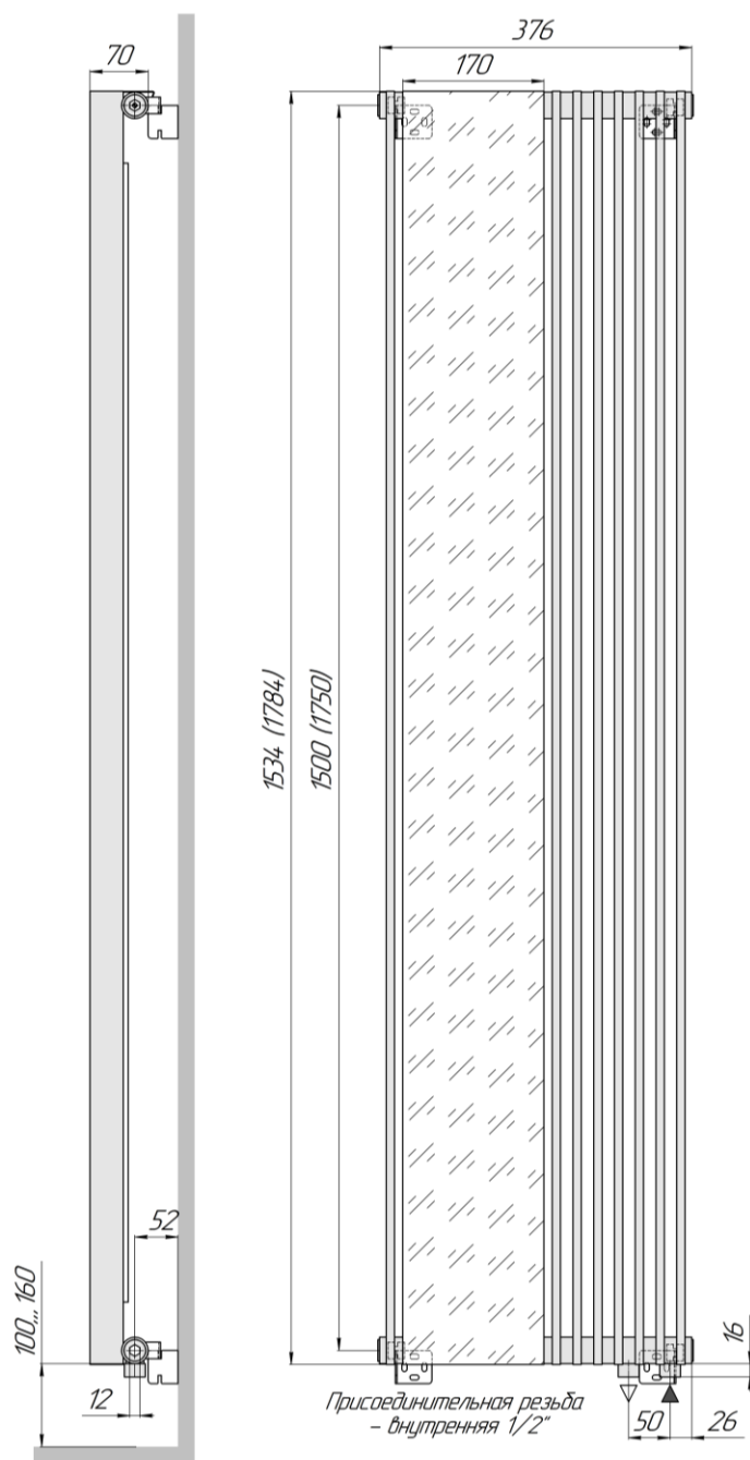
Зеркало П 1-1-7 (вид сбоку, кронштейны КС 22)
