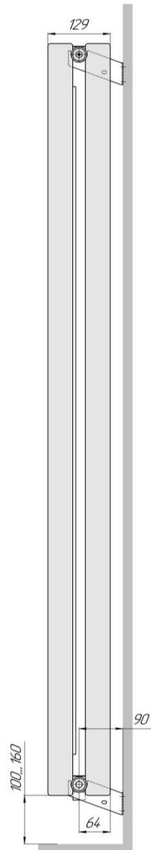
Зеркало 2-3-3 (вид сбоку, кронштейны Г 90)
