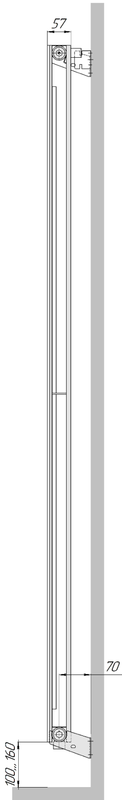
Зеркало С 2 (вид сбоку)
