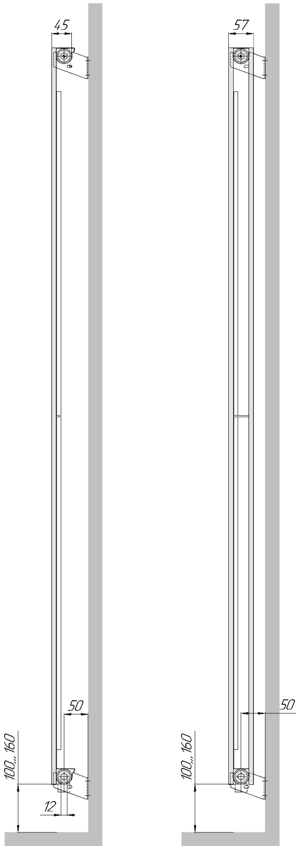
Зеркало С 1-3-3 (вид сбоку, кронштейны С 50)
