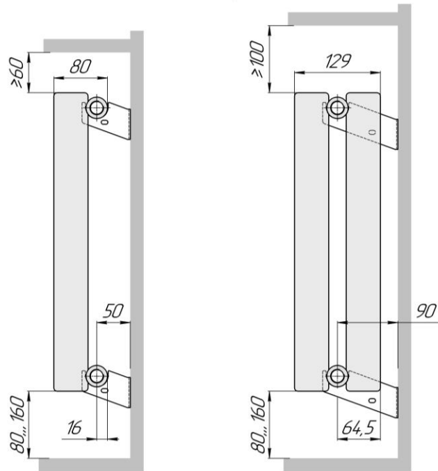
Гармония 1 (вид сбоку, кронштейны Г 50)
