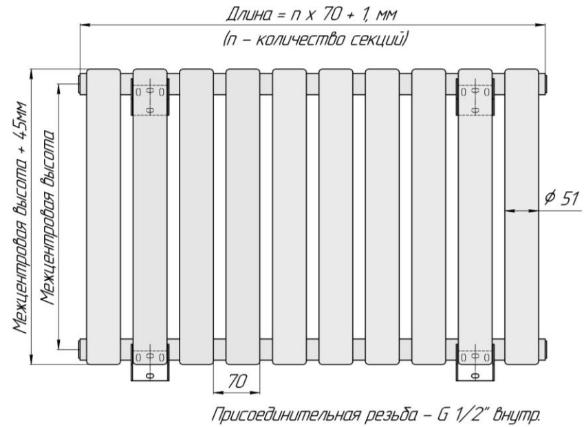
Гармония 1 (вид сверху)
