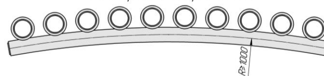
Гармония 1 нп Rнаружн. (вид сверху, изготавливается без встроенного термоклапана)
