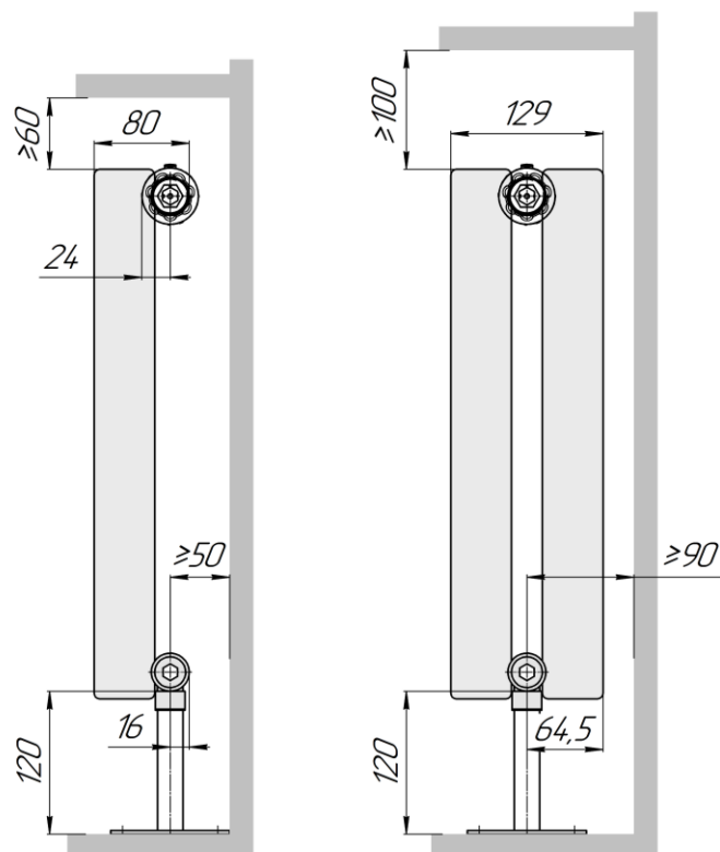
Гармония 1 нп нв (вид сбоку)
