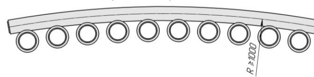
Гармония 1 нп Rнаружн. (вид сверху, изготавливается без встроенного термоклапана)
