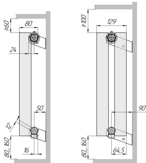
Гармония 1 нп (вид сбоку, кронштейны Г 50)
