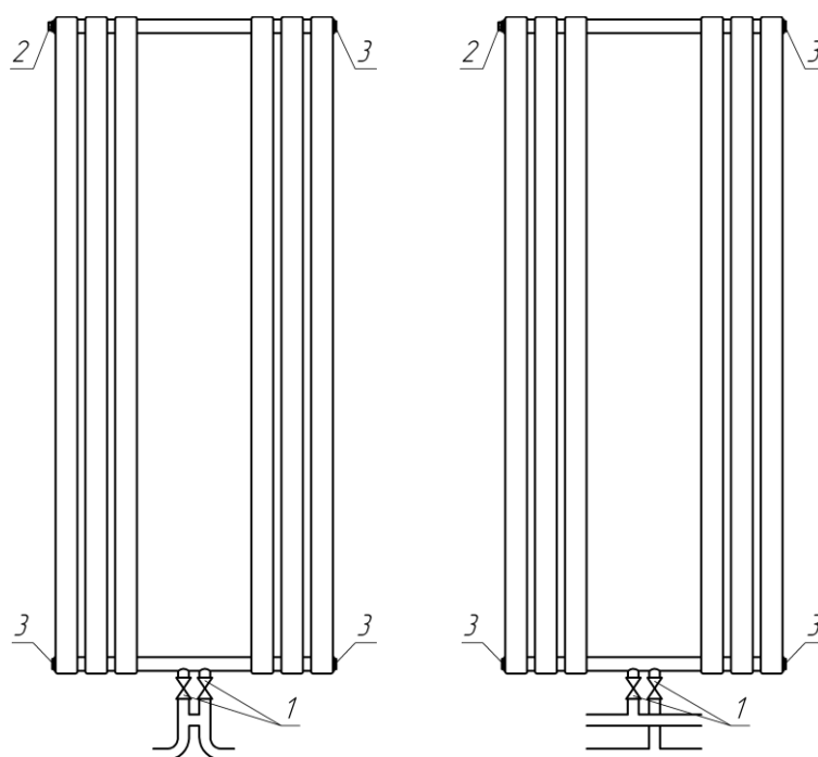
Рис.2 Схема подключения.
