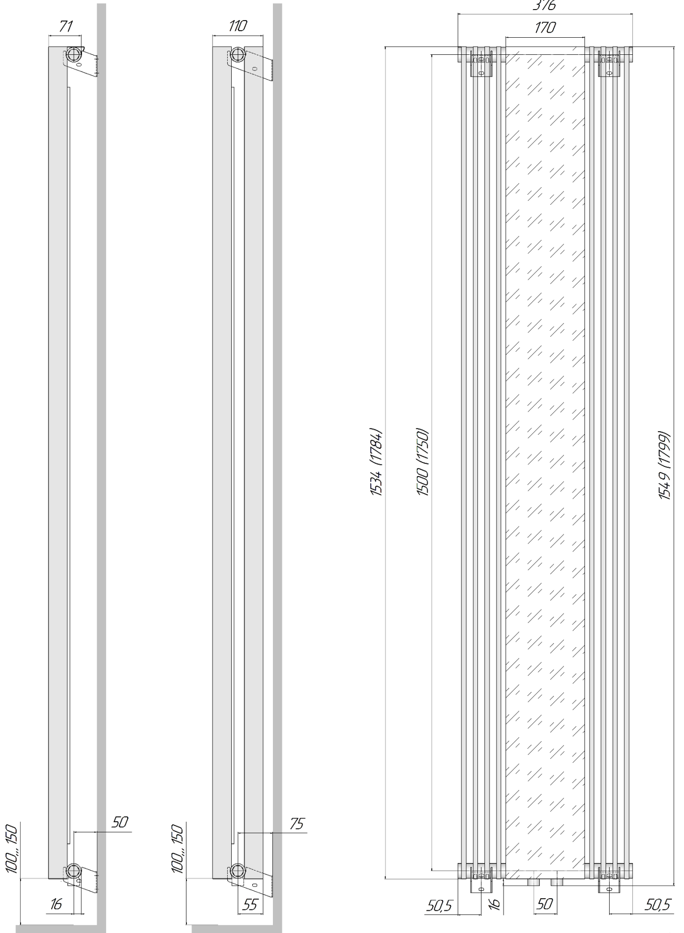
Зеркало П 1-4-4 (вид сбоку, кронштейны С 50)
