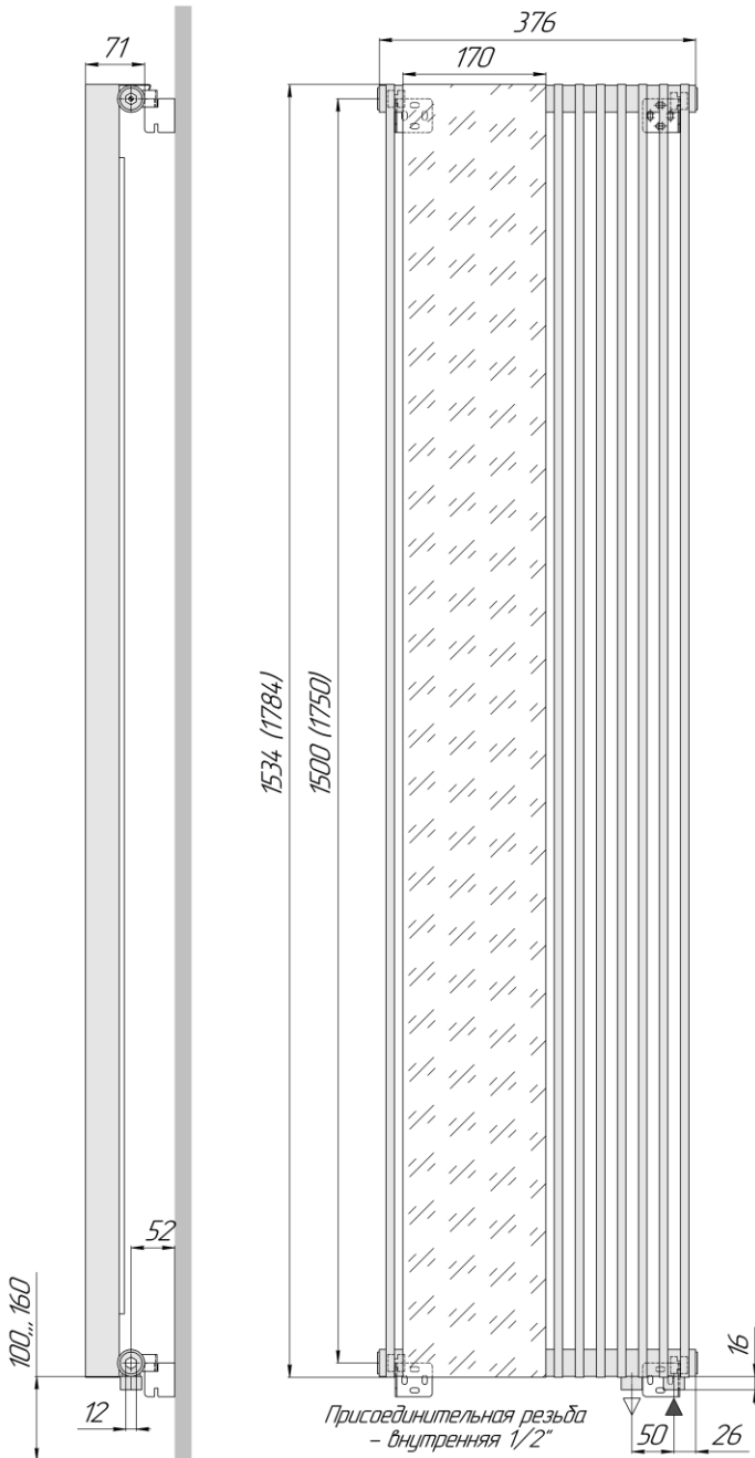
Зеркало П 1-1-7 (вид сбоку, кронштейны КС 22)
