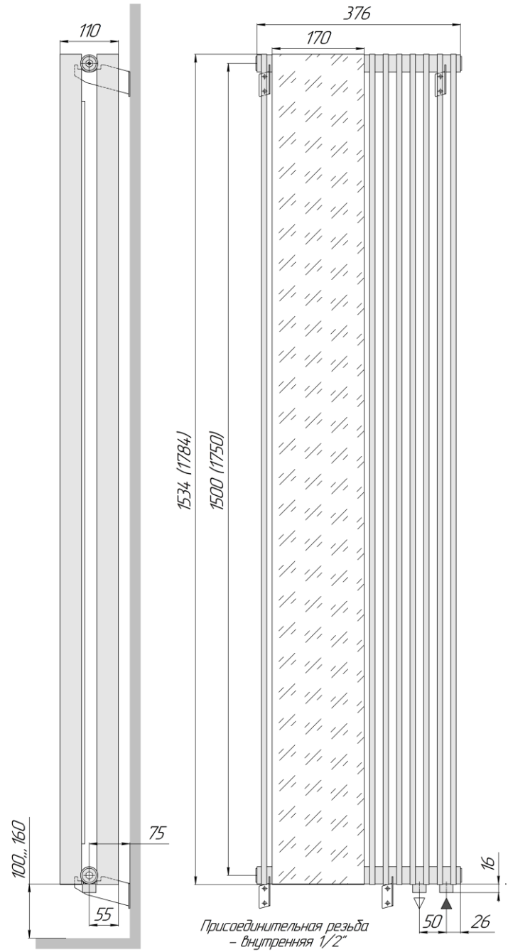
Зеркало П 2-1-7 (вид сбоку, кронштейны КР-2 75)
