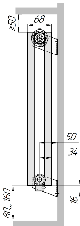
Гармония А20 2 нп (вид сбоку, кронштейны Г 50)
