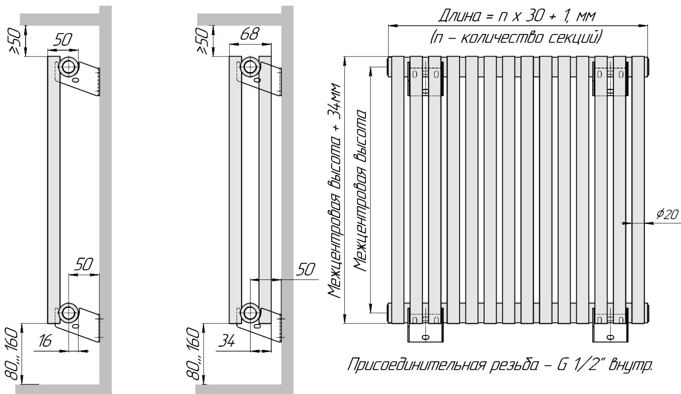
Гармония А20 1 (вид сбоку, кронштейны Г 50) Гармония А20 2 (вид сбоку, кронштейны Г 50)
