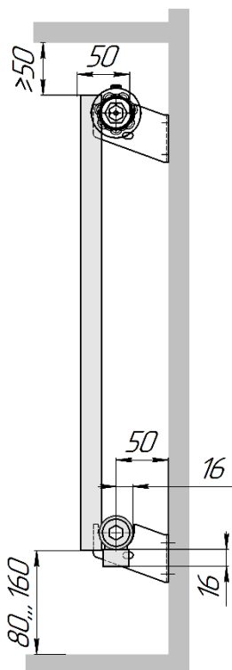
Гармония А20 1 нп (вид сбоку, кронштейны Г 50)
