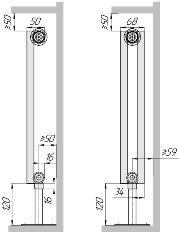
Гармония А20 1 нп нв (вид сбоку)
