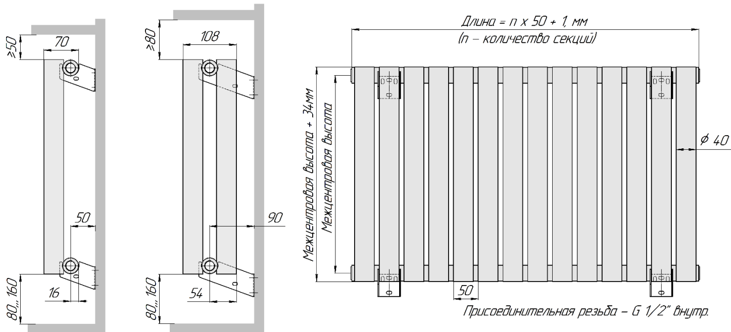
Гармония А40 1 (вид сбоку, кронштейны С 50)
