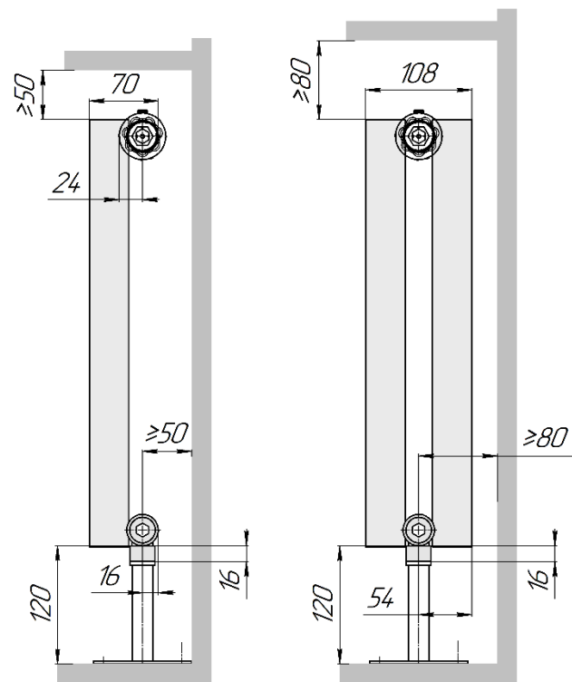
Гармония А40 1 нп нв (вид сбоку)
