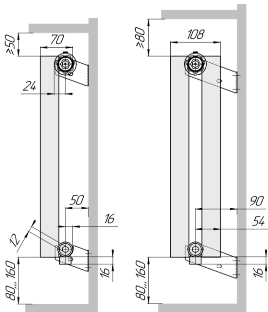
Гармония А40 1 нп (кронштейны С 50)
