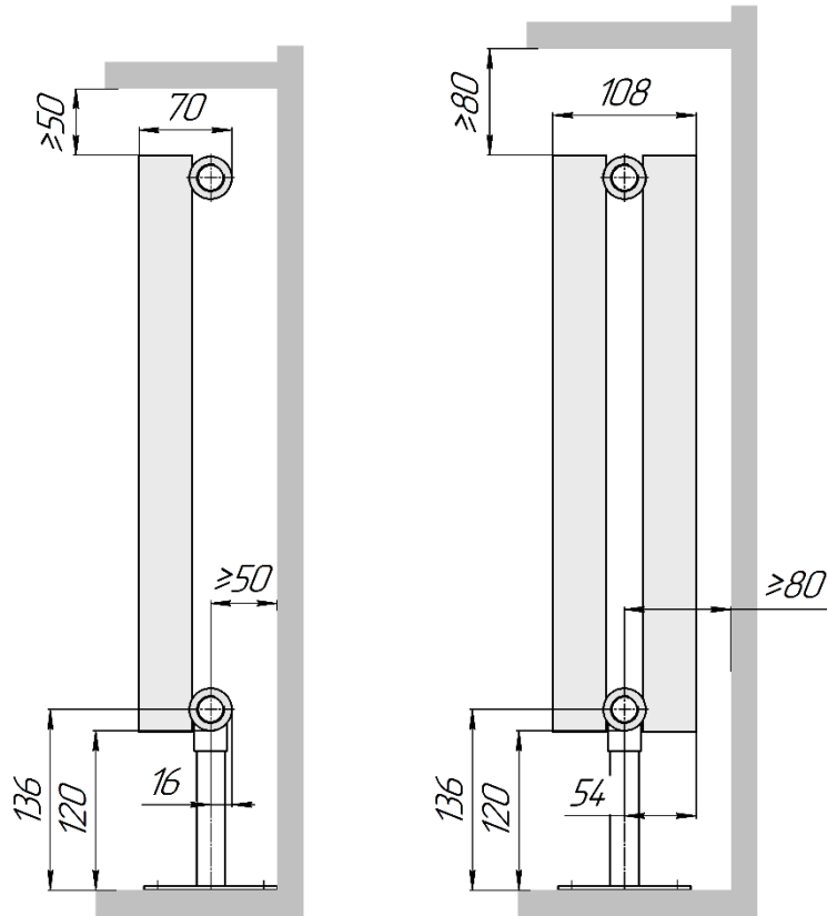
Гармония А40 1 нв (вид сбоку)
