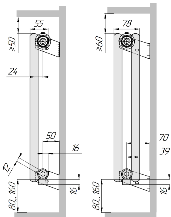
Гармония С25 N 1 нп (вид сбоку, кронштейны К 50)
