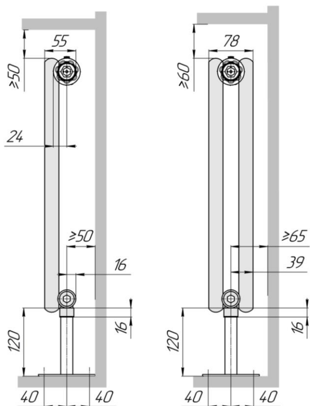
Гармония С25 N 1 нп нв (вид сбоку)
