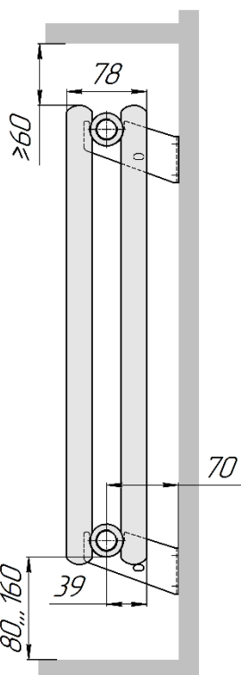
Гармония С25 N 2 (вид сбоку, кронштейны К 70)
