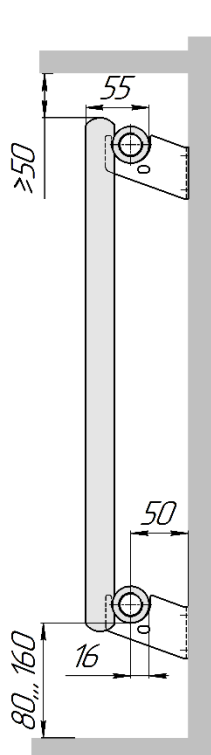
Гармония С25 N 1 (вид сбоку, кронштейны К 50)
