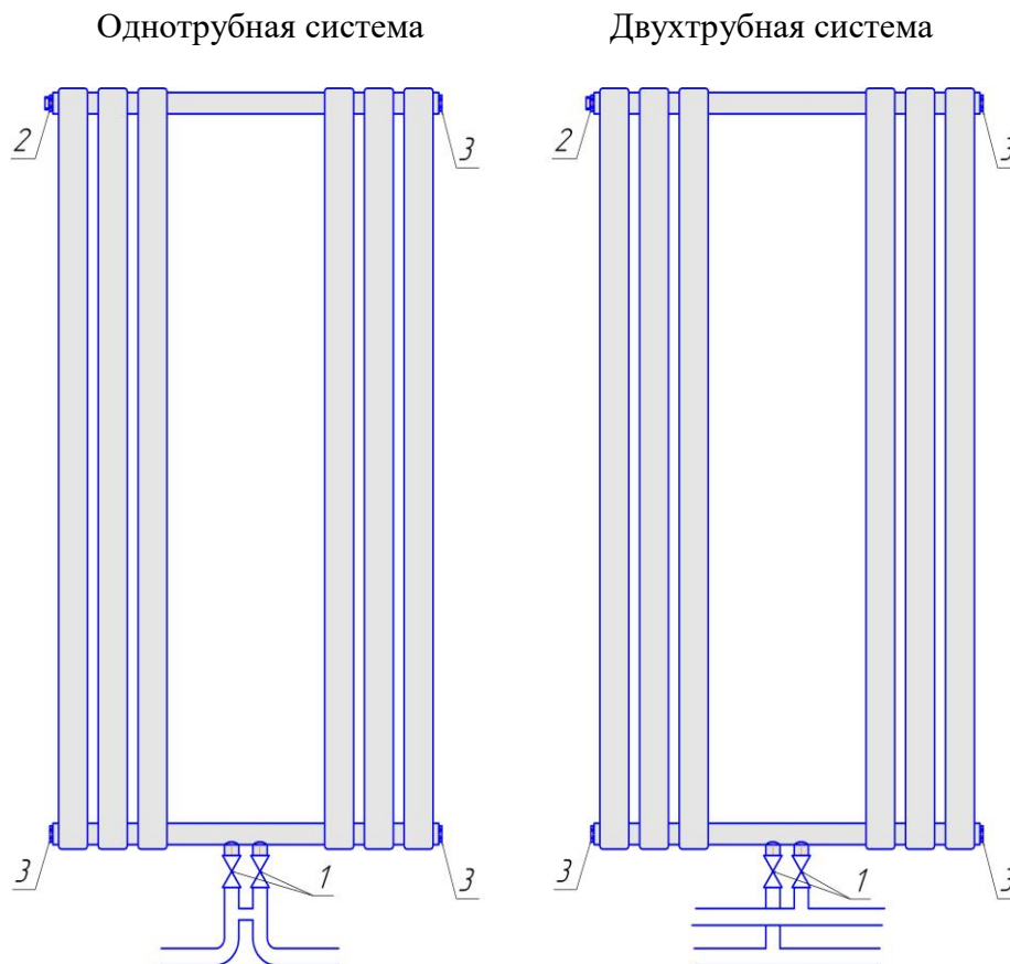
Рис.2 Схема подключения.
