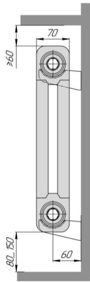
BATARIA 2 кронштейны Б 60
