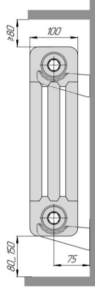
BATARIA 3 кронштейны Б 75
