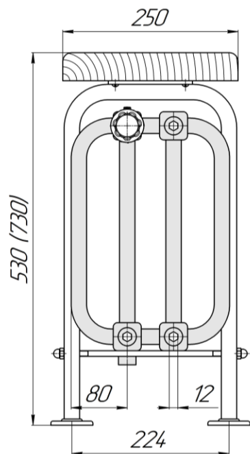
Радиатор напольный с нижним правым подключением "Завалинка РС нп прав" с встроенным термоклапаном, монтажная схема (левое нижнее подключение - зеркально)
