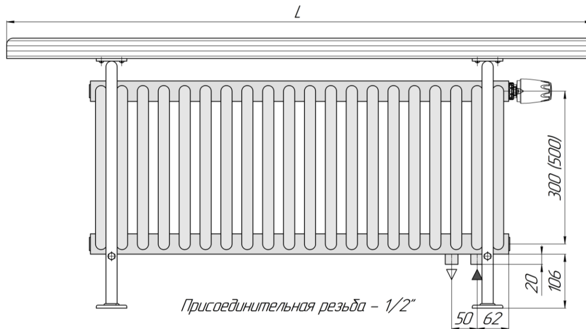
Радиатор напольный с нижним правым подключением "Завалинка РС нп прав" с встроенным термоклапаном, монтажная схема (левое нижнее подключение - зеркально)
