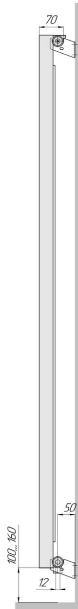
Зеркало А40 1-3-3 (вид сбоку, кронштейны С 50)
