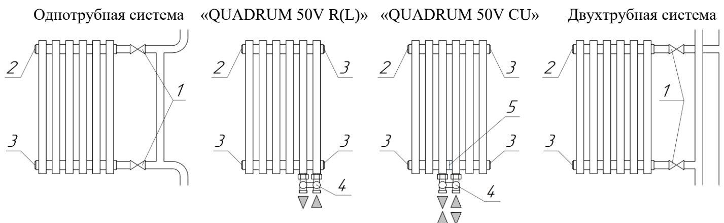
Рис. 2 1. Вентиль. 2. Кран Маевского - воздухоотводчик. 3. Пробка глухая. 4. Запорно-присоединительный клапан нижнего подключения. 5. Внутренняя перегородка.
