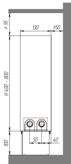
Исполнение "нв" (нерегулируемая высота)
