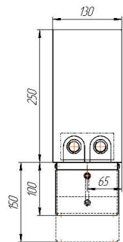
Исполнение "рв" (регулируемая высота)
