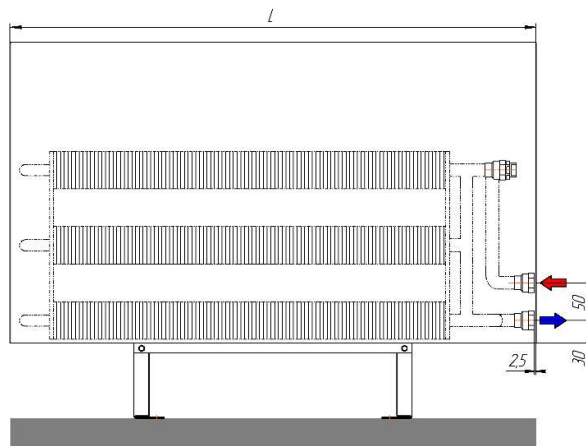
Монтажная схема напольного конвектора "Элегант – плюс 130xH-3то бок нв (рв)" с боковым подключением (присоединительная резьба - 1/2" внутр.)
