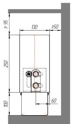
Исполнение "нв" (нерегулируемая высота)
