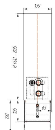
Исполнение "рв" (регулируемая высота)
