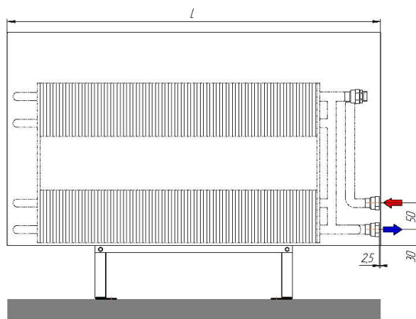
Монтажная схема напольного конвектора "Элегант – плюс 130xH-4то бок нв (рв)" с боковым подключением (присоединительная резьба - 1/2" внутр.)
